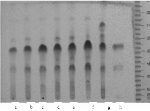
a ~ c. 3 批独一味水提物;d ~ f. 3 批止血镇痛散; g. 对照药材;h. 对照品溶液
